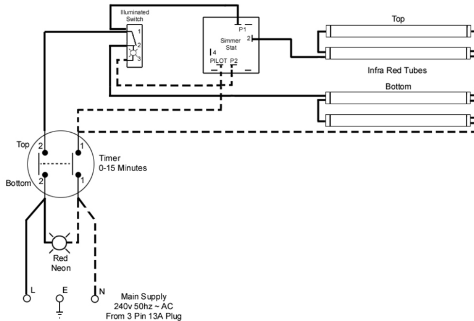
CAS Wiring Diagram
