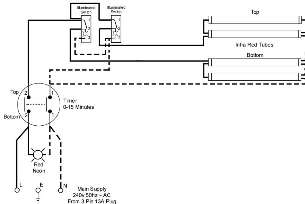
CPG Wiring Diagram
